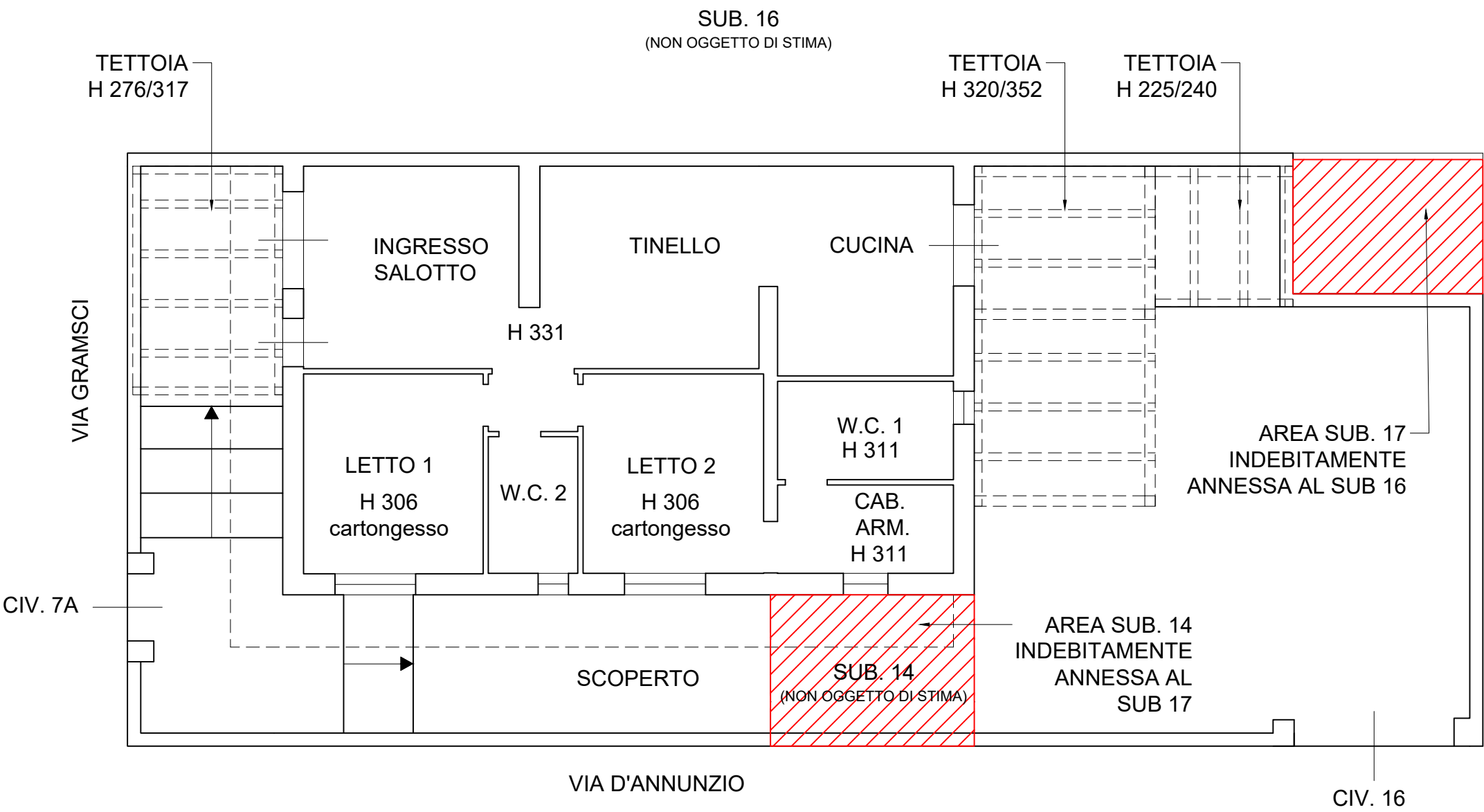
PLANIMETRIA STATO DEI LUOGHI SUB. 17 - PIANO TERRA - SCALA 1:100
